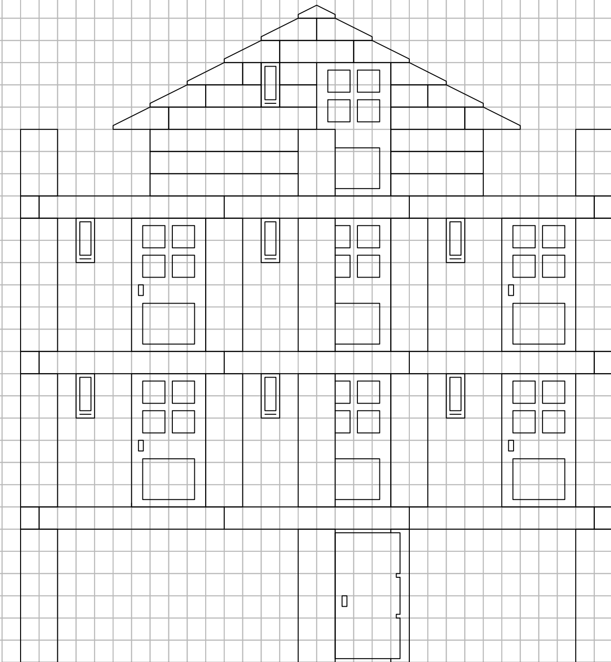
AANZICHT - ACHTERZIJDE
